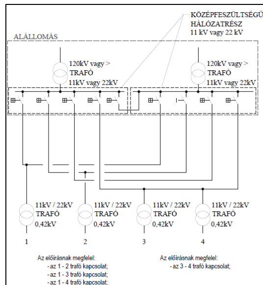
6. ábra Biztonsági tápellátás megvalósítása közüzemi villamos hálózatról
