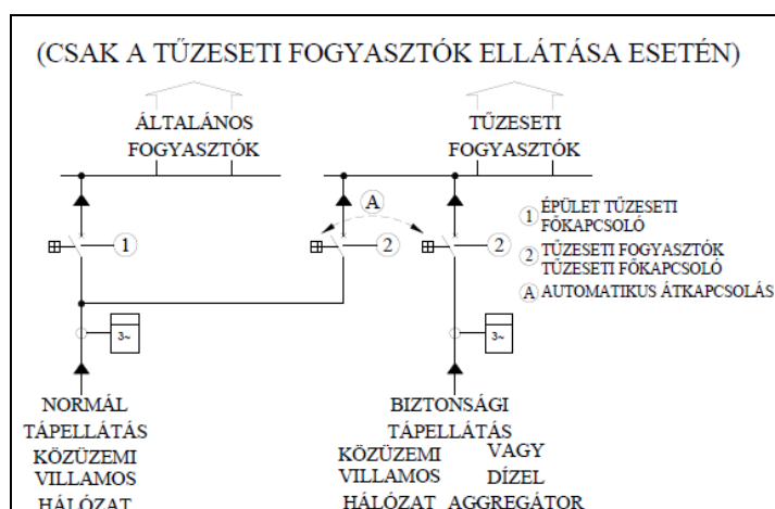
8. ábra Tűzeseti fogyasztók ellátás kettős biztonságú betáplálással „B”
