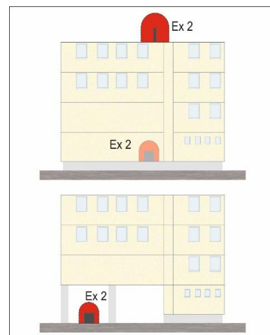
15. ábra: Korlátozott mértékű robbanásveszélyes épületek
