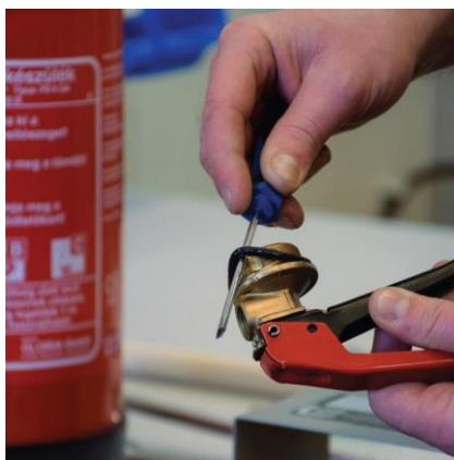
O-gyűrű eltávolítása
